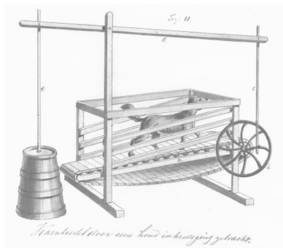
De tekening van de hondentredmolen.
